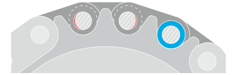
Durch den Verschleiß an den Bolzen und in den Hülsen längt sich die Steuerkette. Im Dauerversuch wurde eine Längung um 0,5 % nach 240.000 km ermittelt (Zahnriemen 0,1 %).
