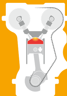
3. Takt (Arbeiten)
