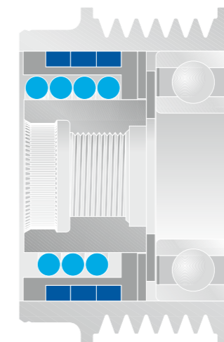
Entkoppelter Generatorfreilauf OAD (Overrunning Alternator Decoupler)
