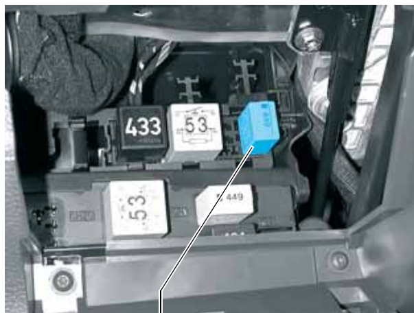
Relais für Kühlmittelzusatzpumpe J496
