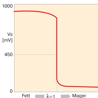
Abb. 3 Ausgangssignal Vs-Signal
