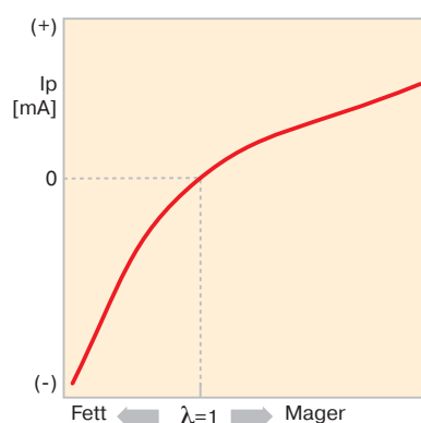
Abb. 4 Ausgangssignal Ip-Signal
